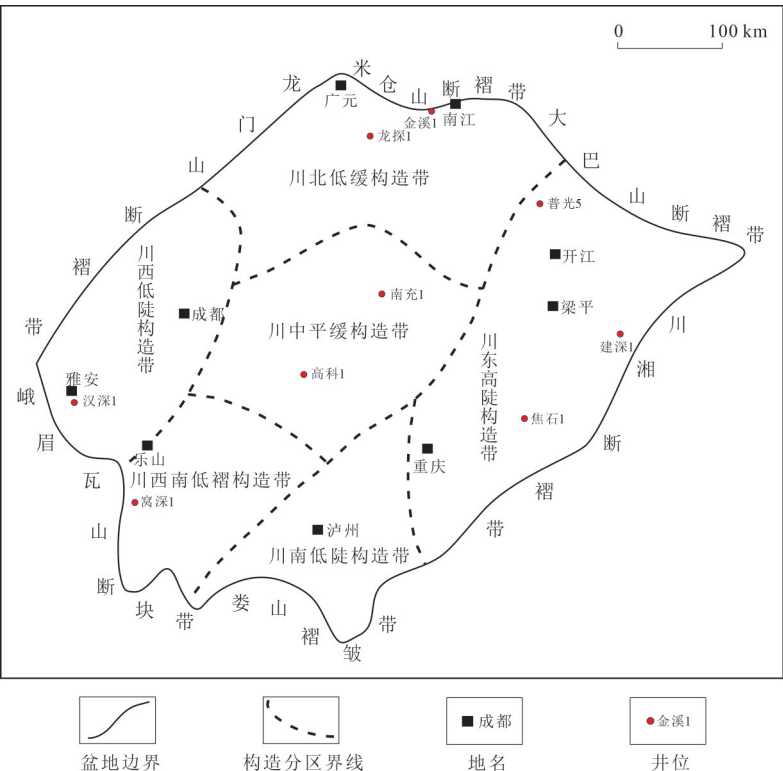
图 1 四川盆地位置及构造单元划分 Fig. 1 Location and tectonic units of the Sichuan Basin
